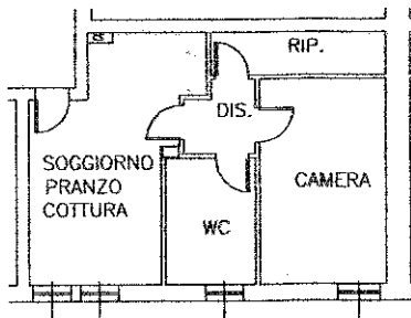
PIANTA PIANO PRIMO H=2.60
